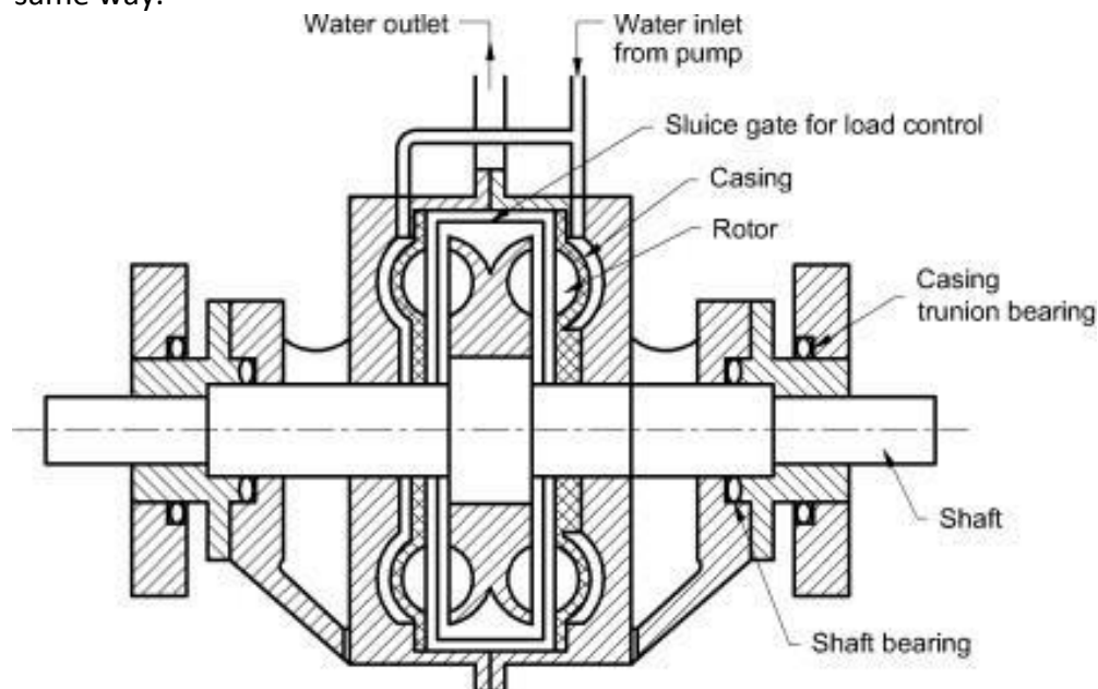
Fig. 9. 5 Hydraulic Dynamometer
