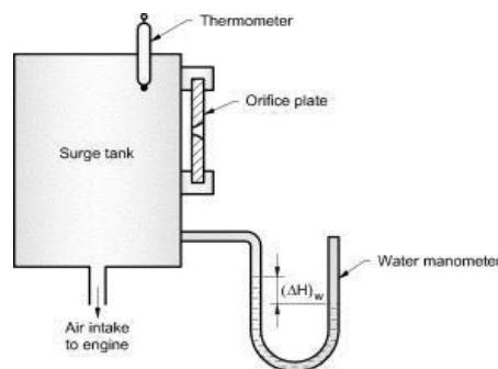
Fig. Air flow meter
