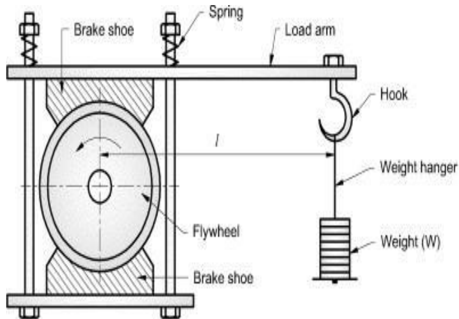
Fig. Prony Brake Dynamometer
