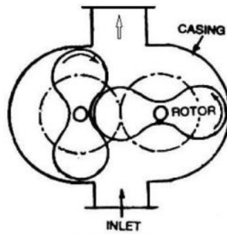
Fig:4.11 Roots blower
