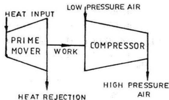
Fig: Air Compressor
