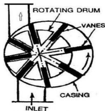
Fig: 4.12 Vane blower
